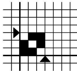
Tejido sarga S 2/1
