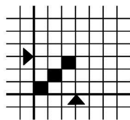
Tejido sarga Z 1/2
