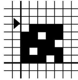
Tejido raso satén (Efecto de urdimbre)
