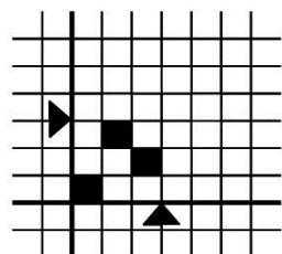
Tejido sarga S 1/2
