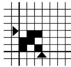
Tejido sarga Z 2/1
