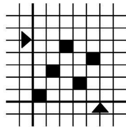
Tejido raso satén (Efecto de trama)
